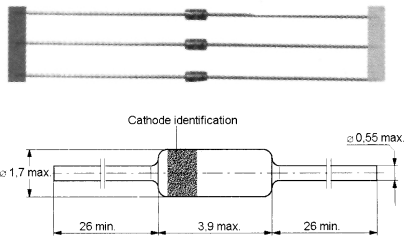
DO35
