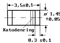
Minimelf
